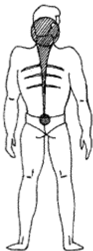
Рис. 96. Программа зомбирования
